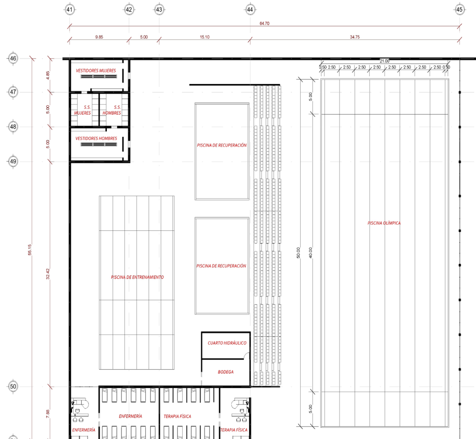
Centro de Natación - Planta
