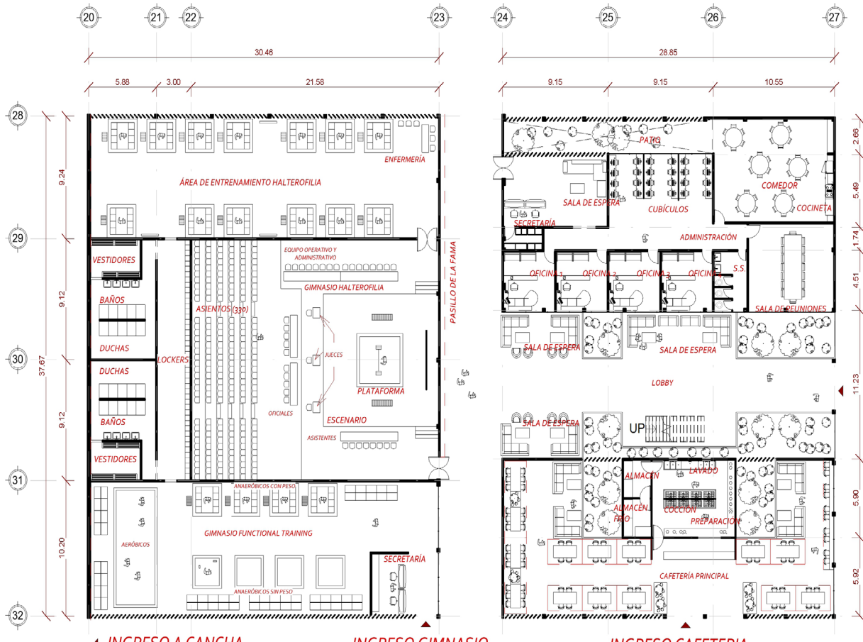
Centro de Halterofilia y Comedor y área común - Planta
