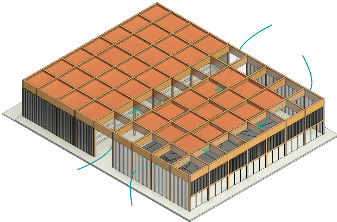
Isometrico Estudio de Ventilación
