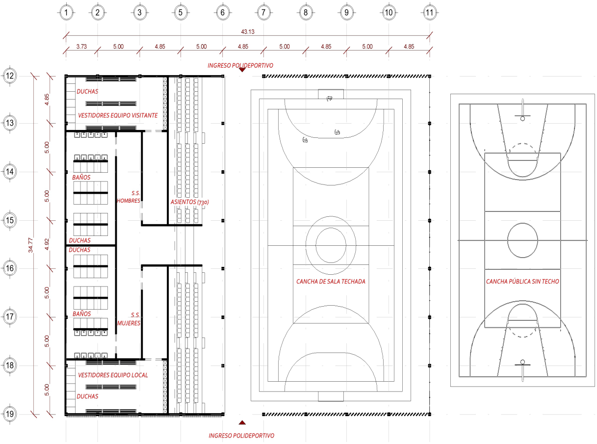
Centro Polideportivo - Planta
