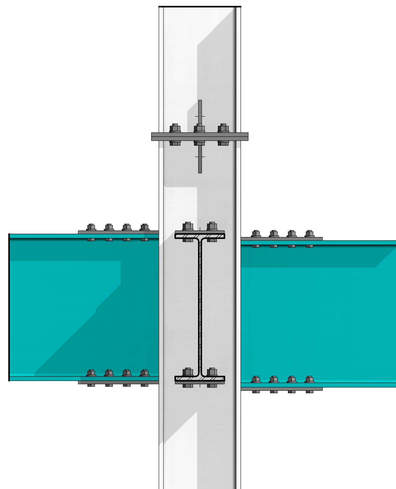
2 Vista frontal conexiones en cruz y columnas empalmadas
