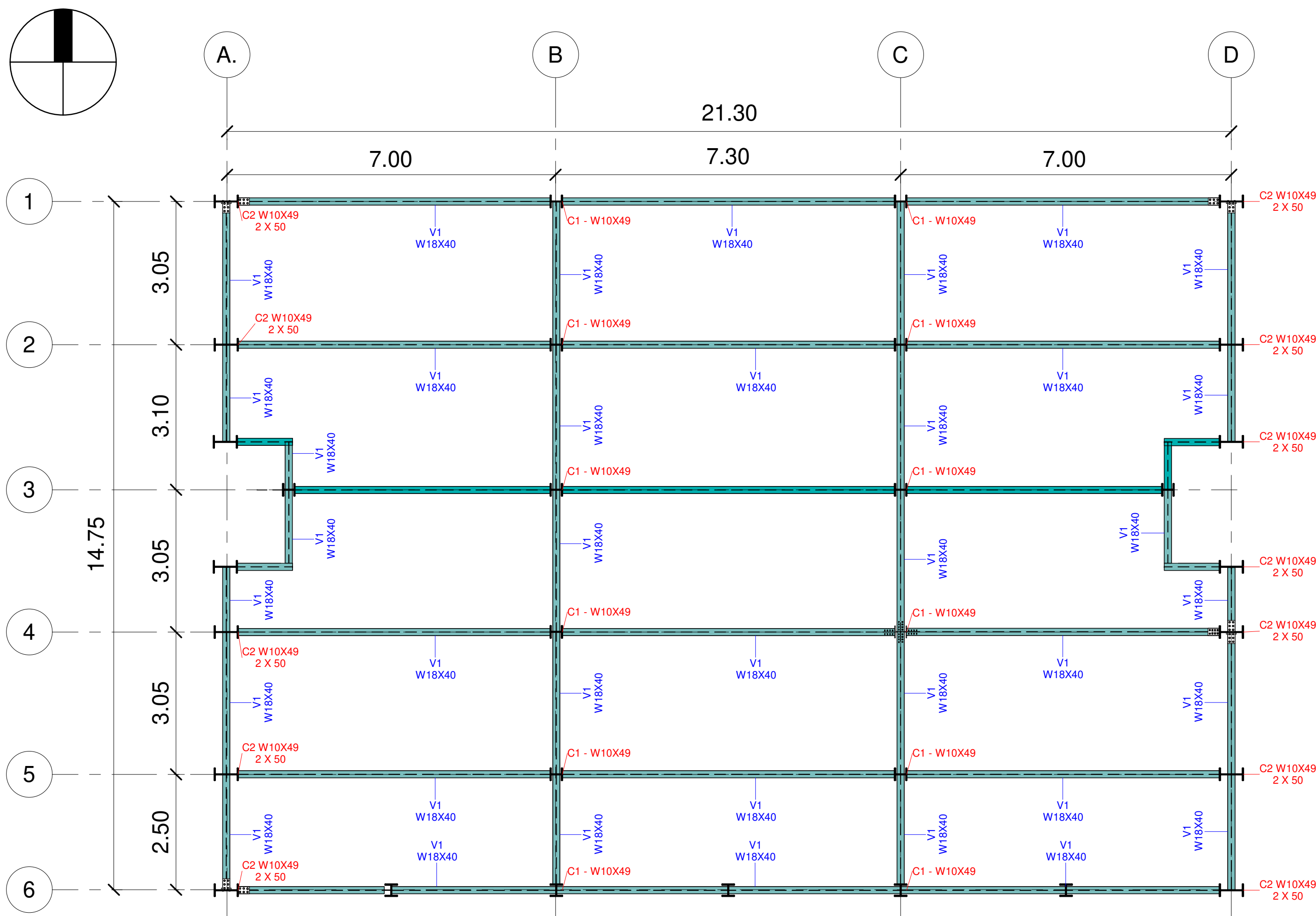
1 Planta Marcos 1 : 75
