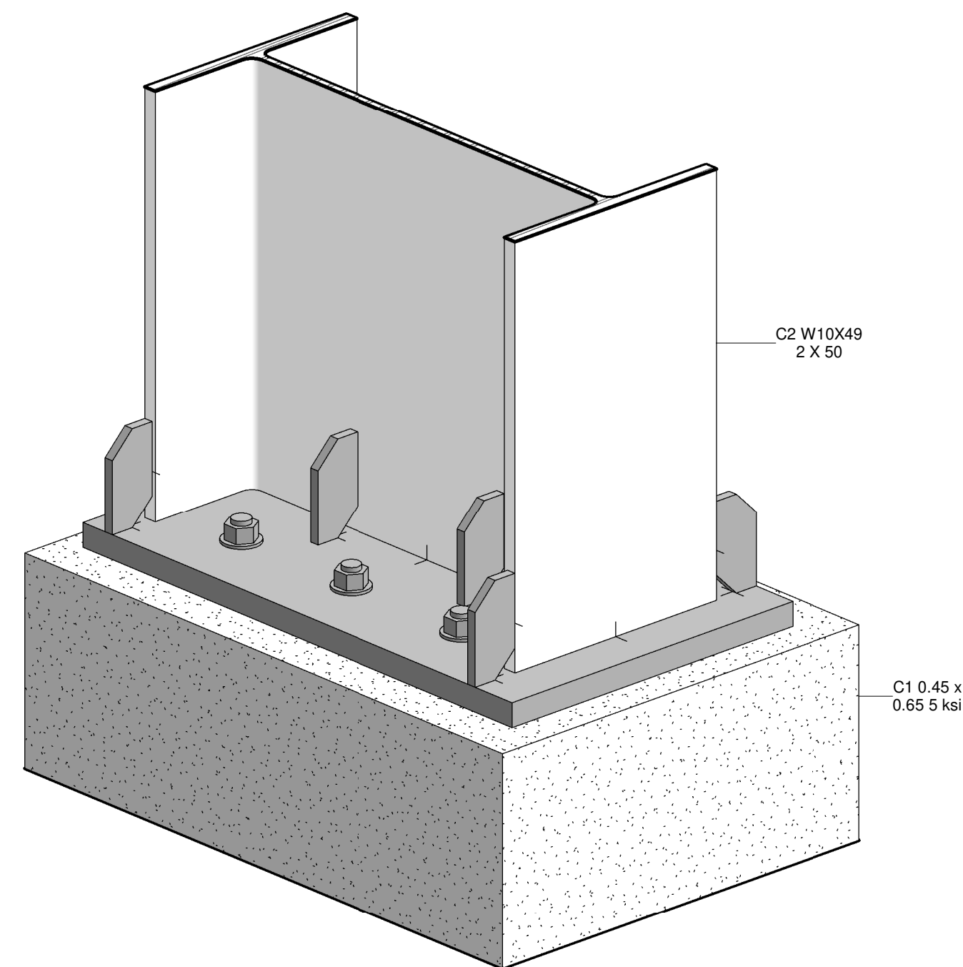
5 PLATINA COLUMNA C1
