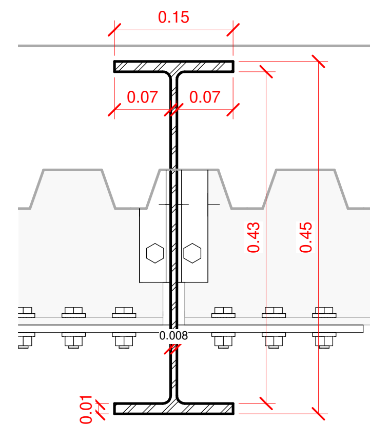
5 Perfil Viga V1 Copia 1 1 : 5
