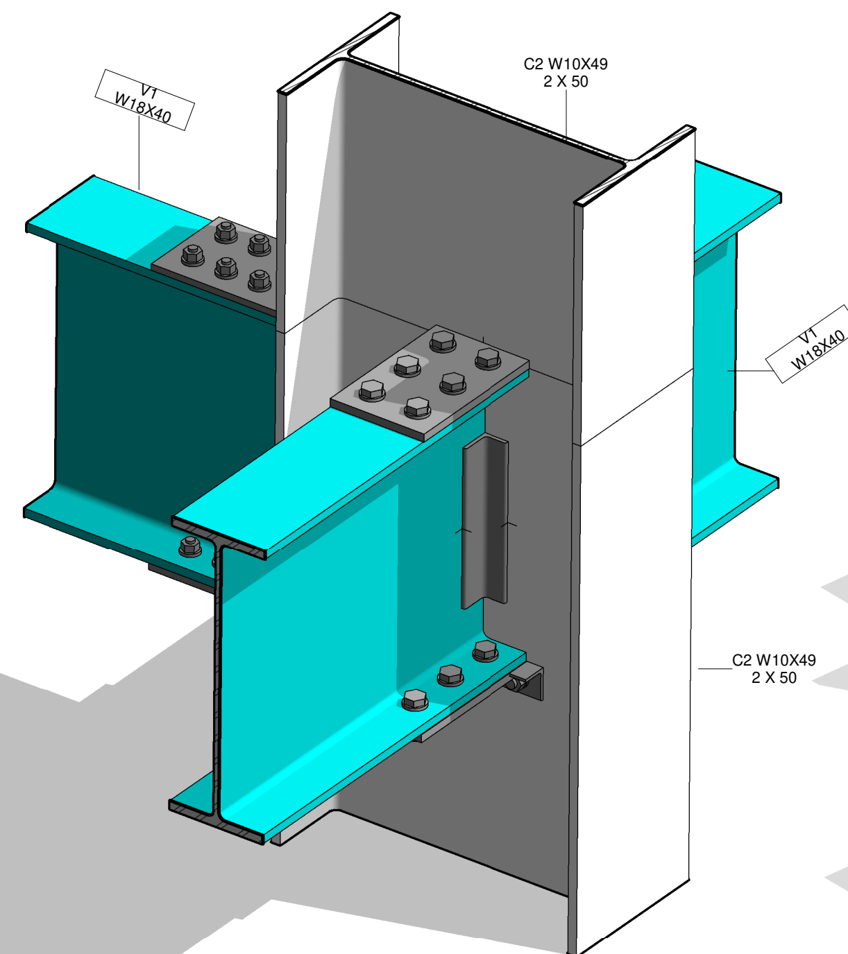
5 Vista conexión en T
