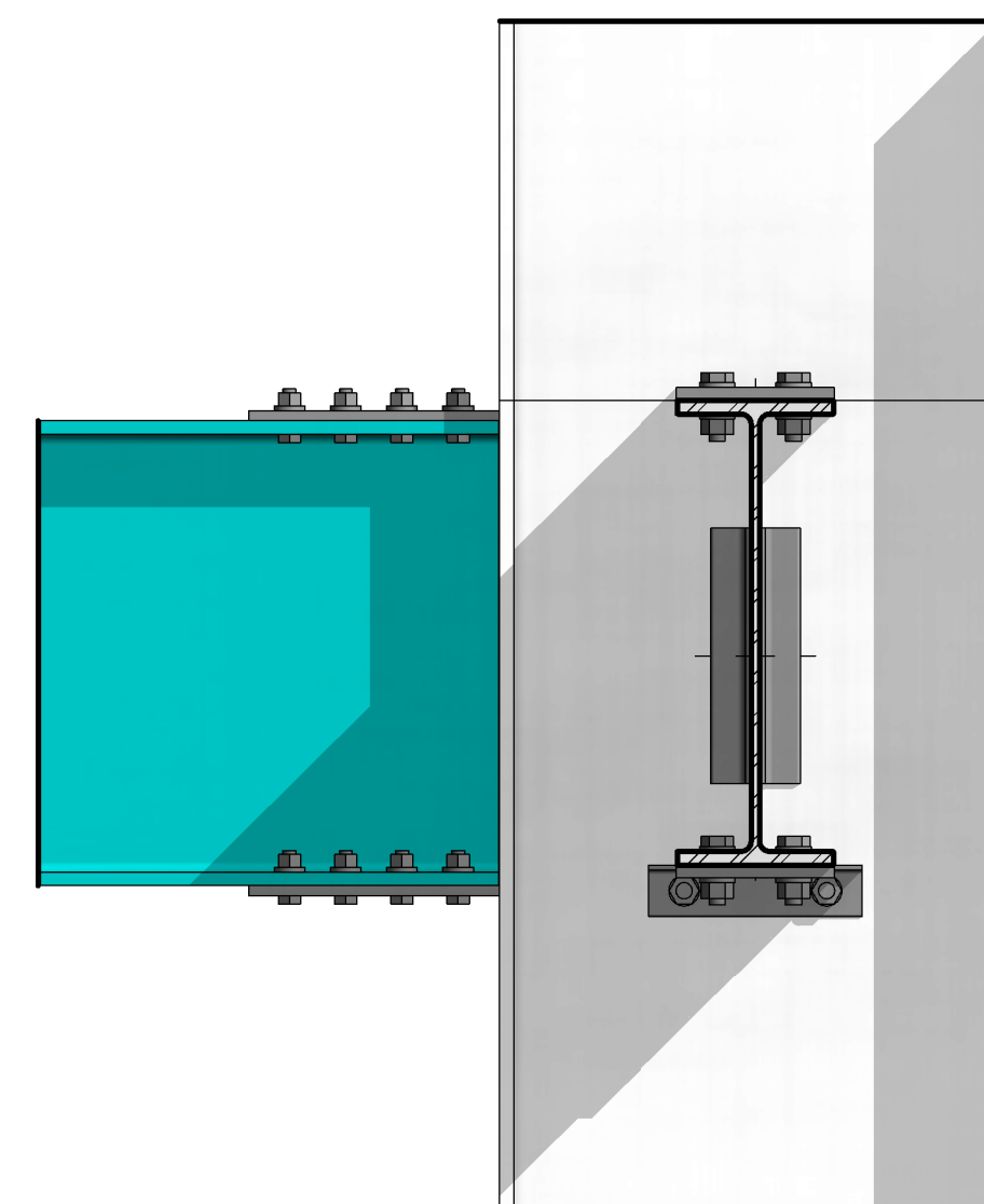
8 Vista frontal conexión en T
