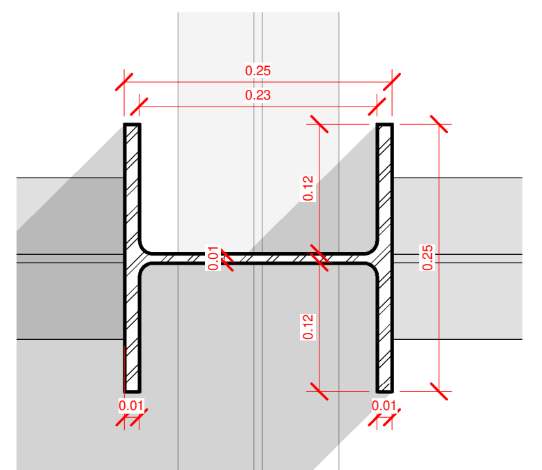
7 Sección Columna C1 1 : 5
