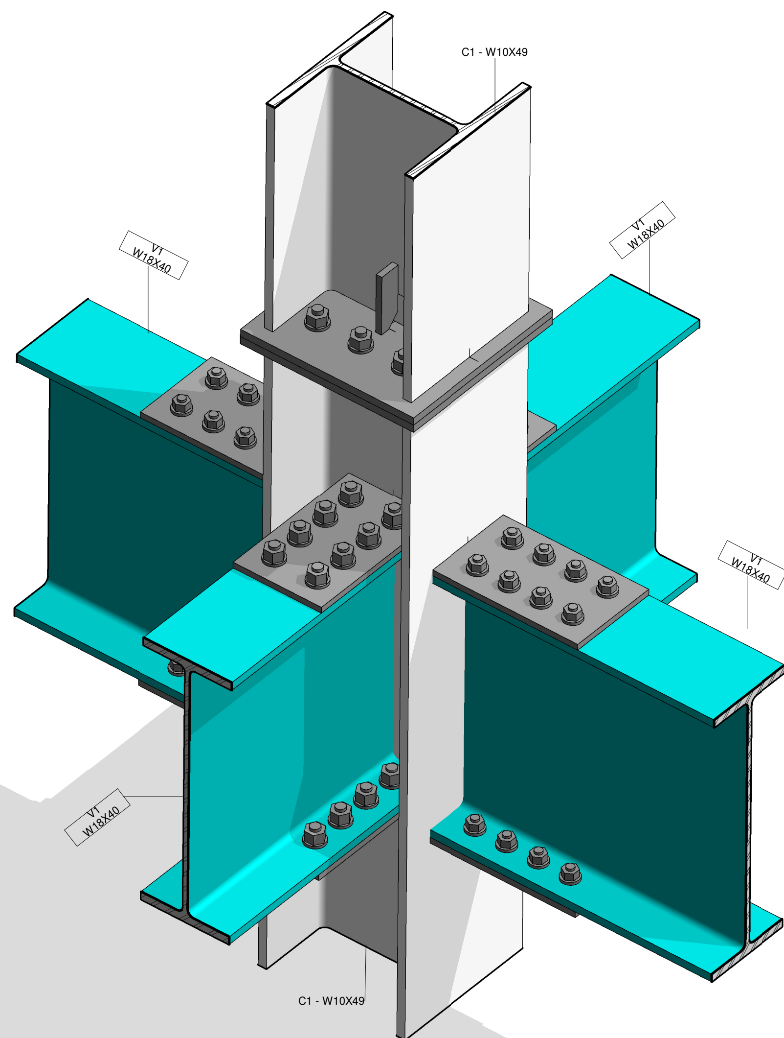
1 Vista conexiones en cruz y columnas empalmadas
