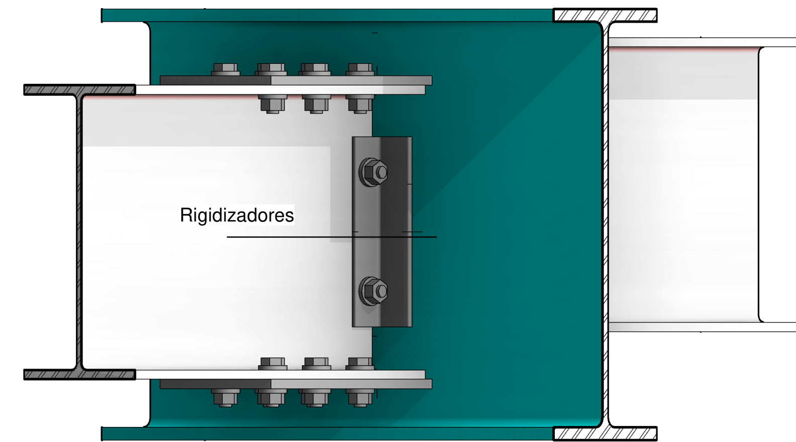
4 Vista de conexión viga secundarias 2
