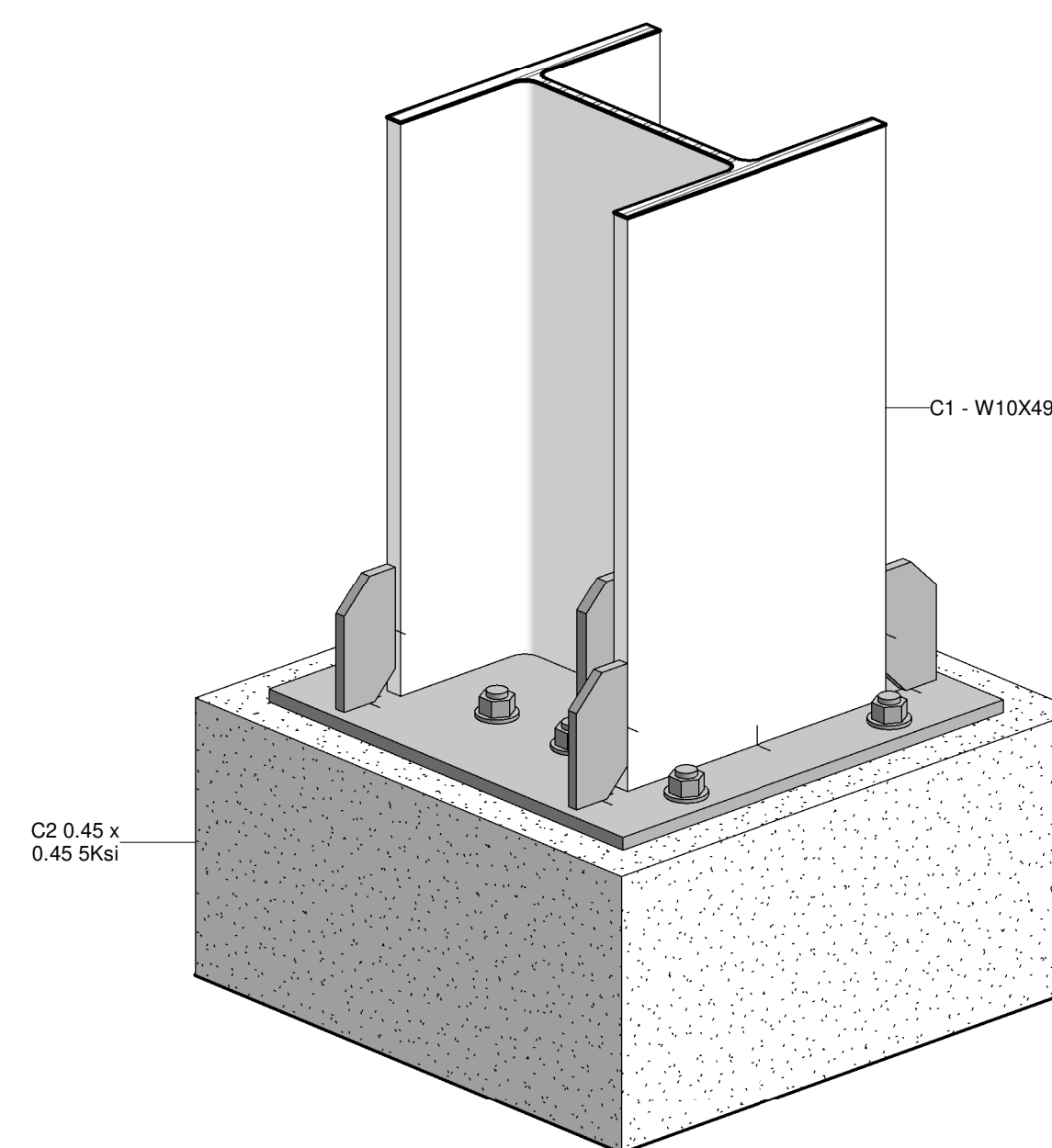
4 PLATINA COLUMNA C2
