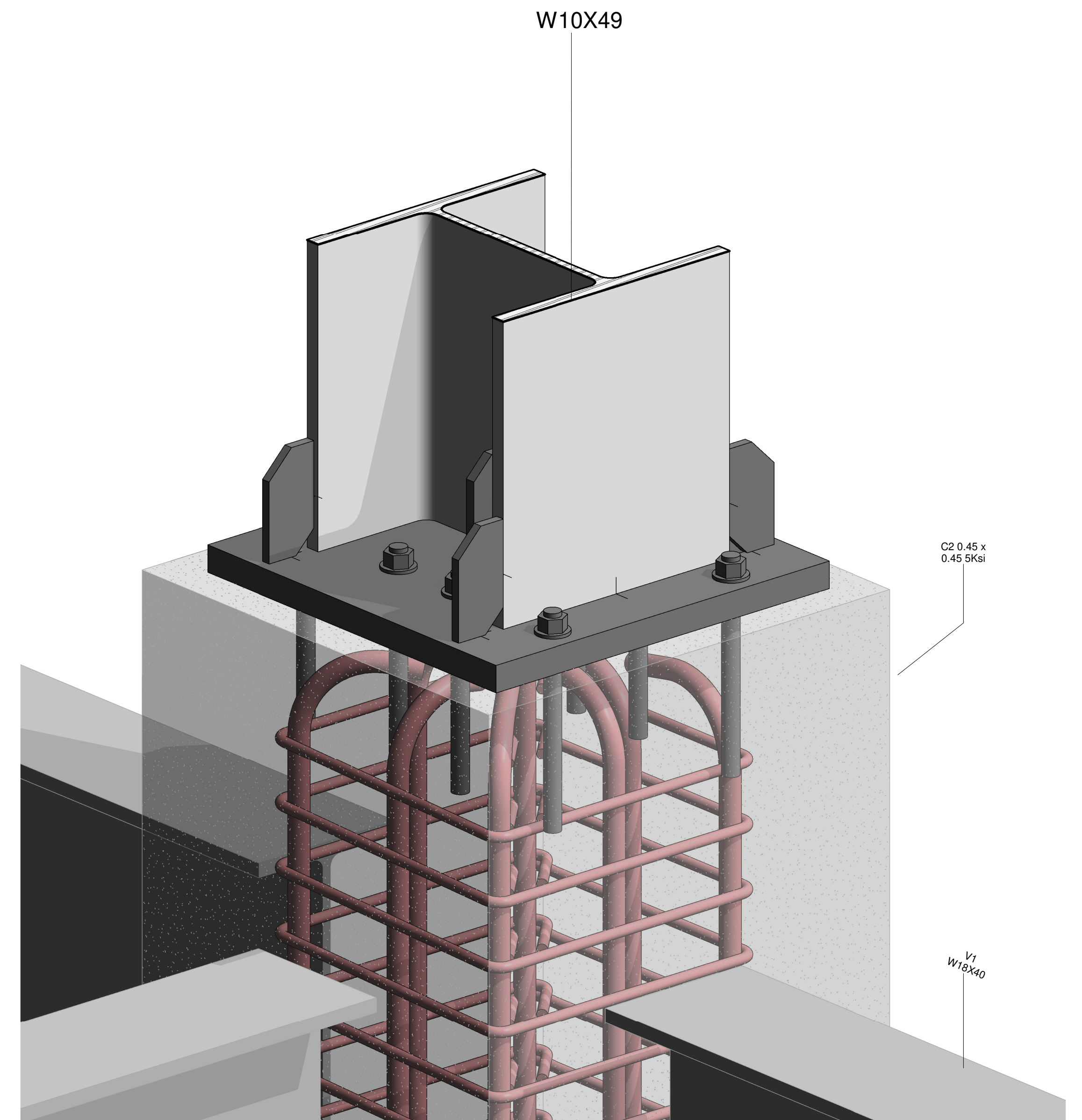
6 Detalle refuerzo de columna y platina
