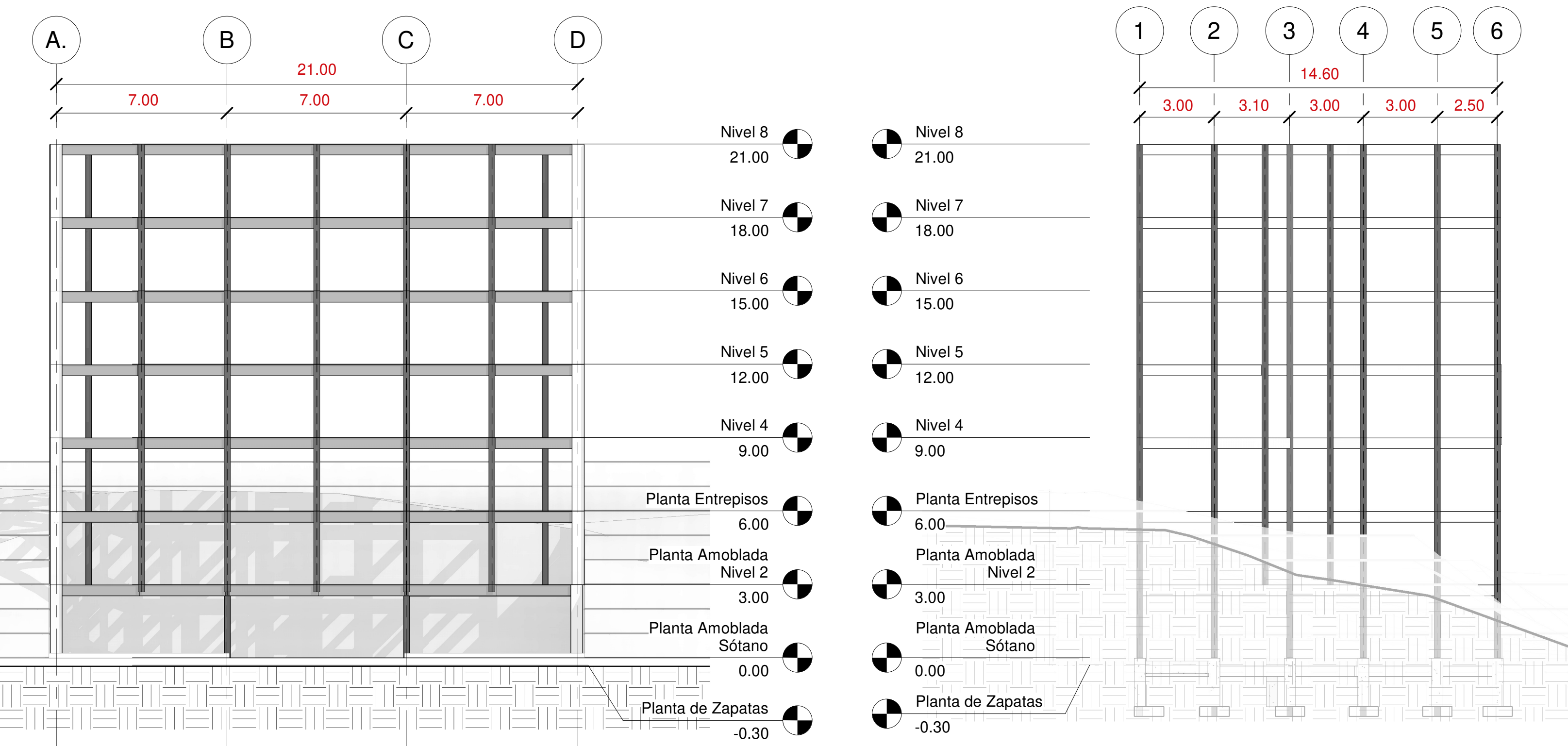
3 Elevación Frontal Marcos 1 : 150
