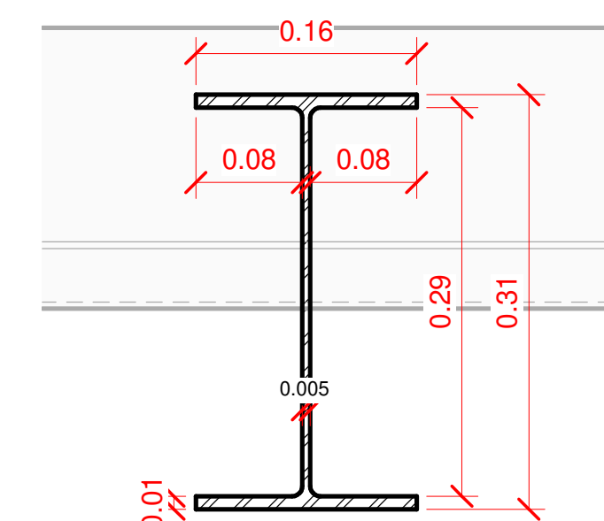
6 Perfil Viga V2 Copia 1 1 : 5
