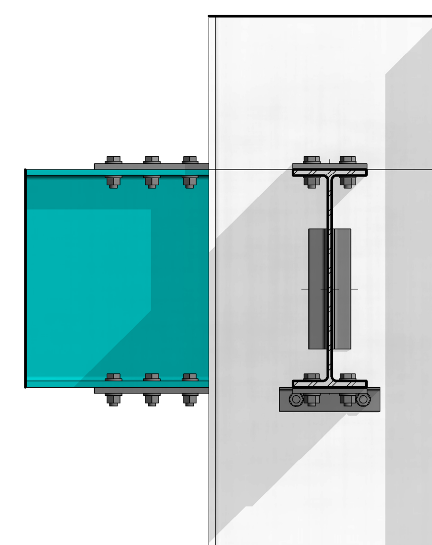
7 Vista frontal conexión en L
