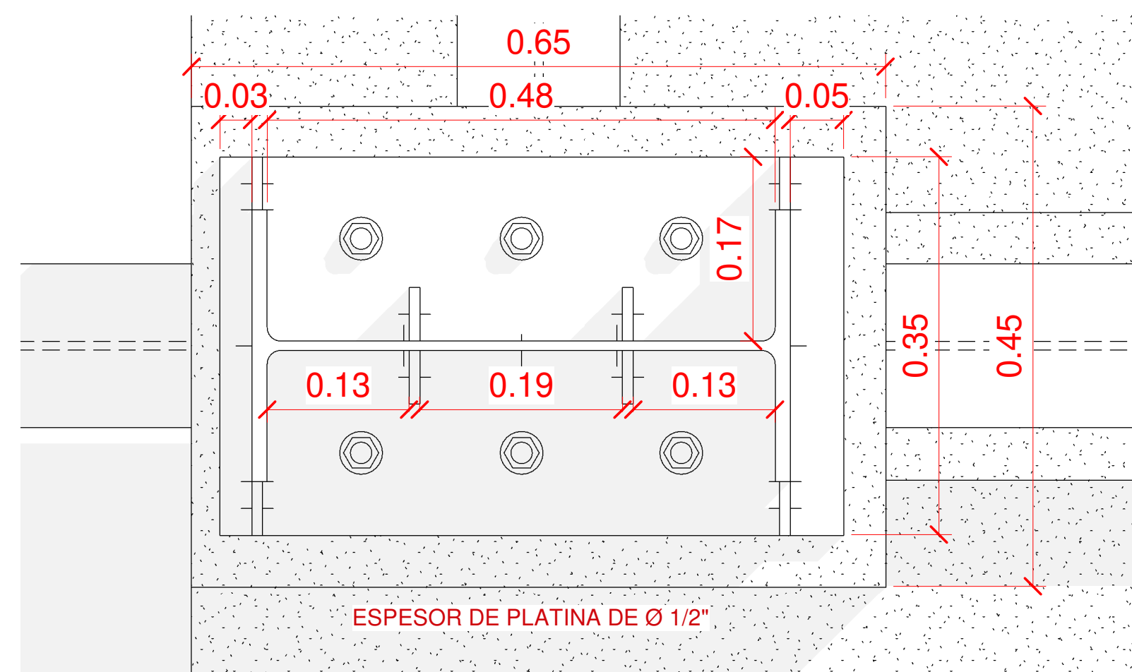
2 Configuración platina para columna C1 1 : 5
