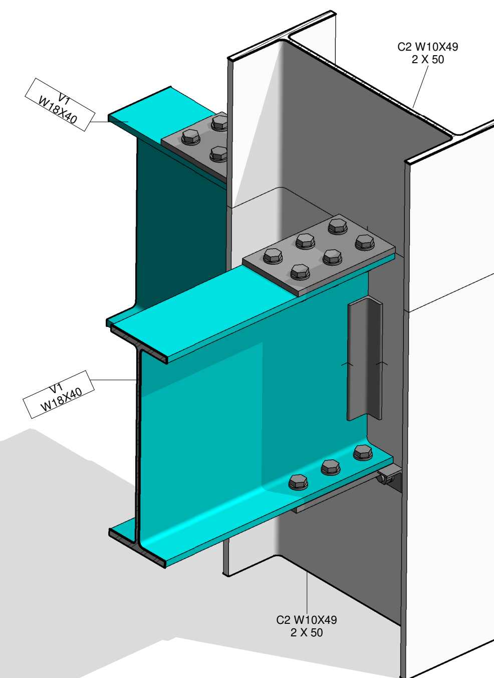
6 Vista conexión en L
