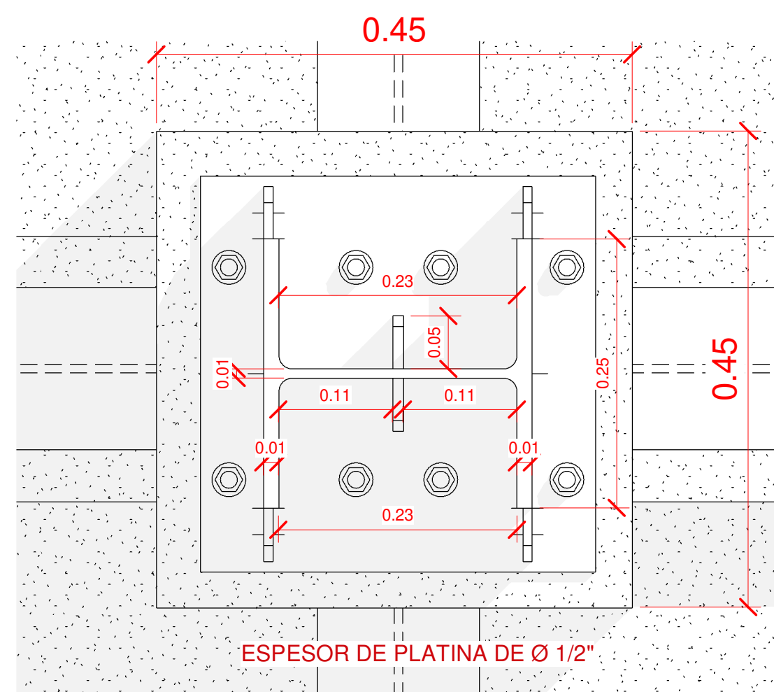
3 Configuración platina para columna C2 1 : 5
