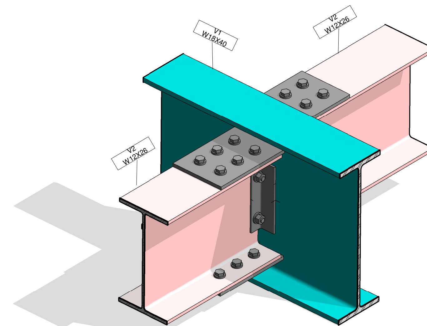
3 Vista de conexión viga secundarias
